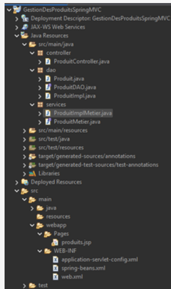
Architecture Maven du projet Spring MVC
